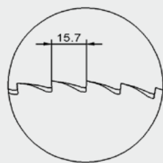
09 Brotmesserverzahnung, 15,7 mm
