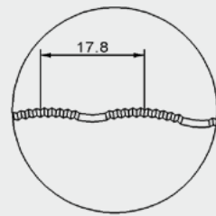
10 Mikroverzahnung, 17,8 mm
