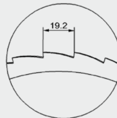
07 Brotmesserverzahnung, 19,2 mm
