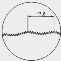
05 Mikroverzahnung konvex, 17,8 mm
