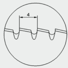
12 Tomatenverzahnung, 4 mm
