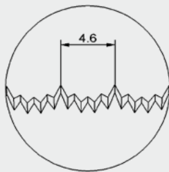
02 Mikroverzahnung konkav, 4,6 mm
